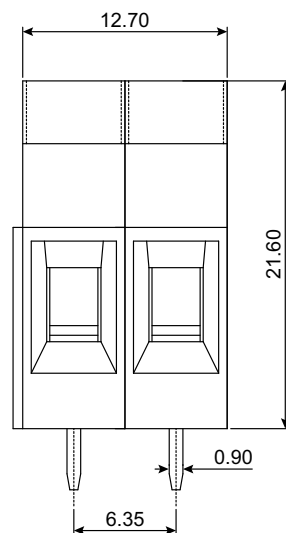
635S 4-way Interlocked
